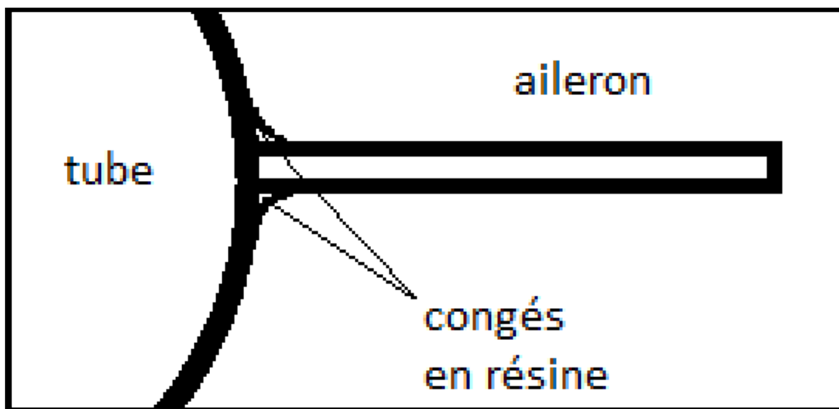
FIGURE 3.2 – Procédé de collage ailerons/structure avec congés en résine
