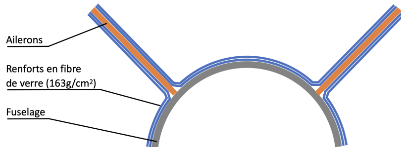
FIGURE 3.3 – Illustration du collage des ailerons sur le tube de la mini-fusée Arcturus .
